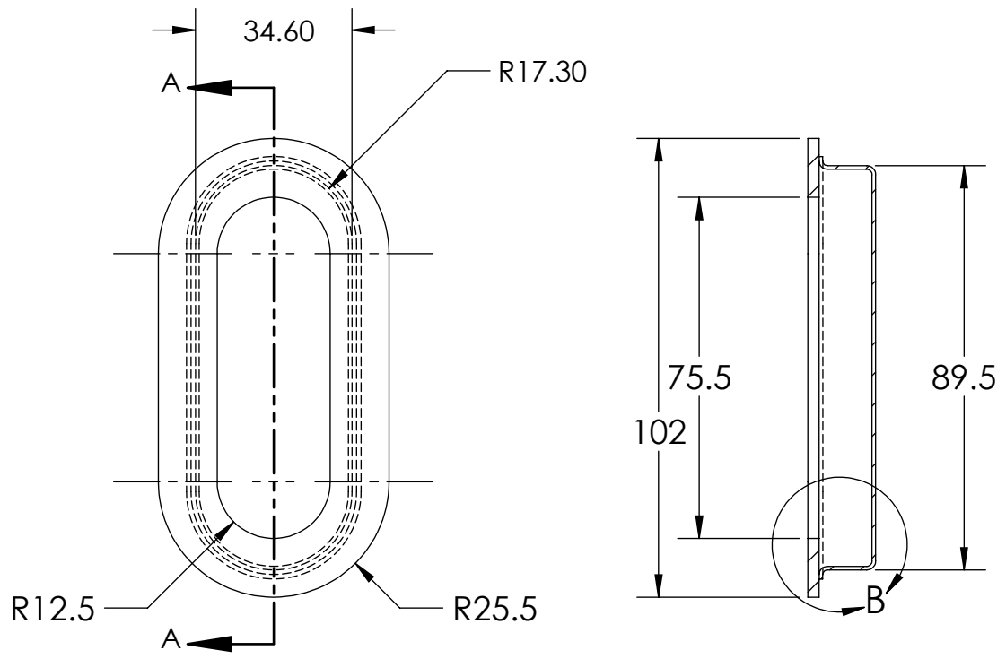
SECTION A-A
