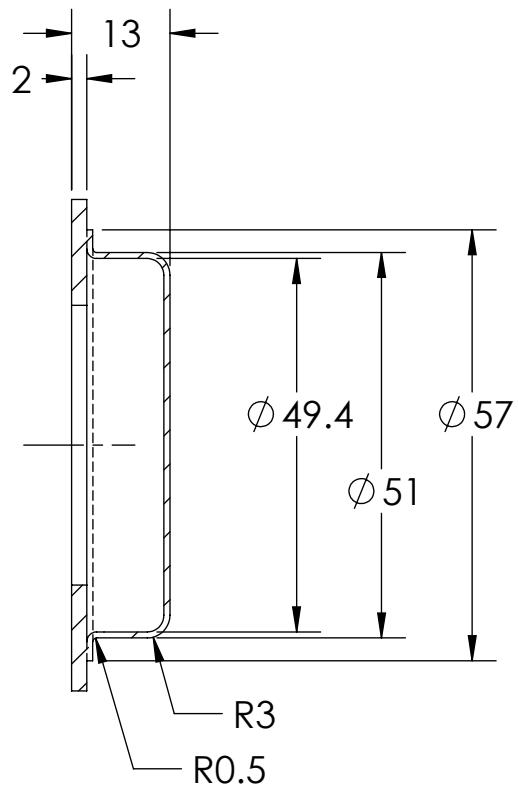
SECTION A-A
