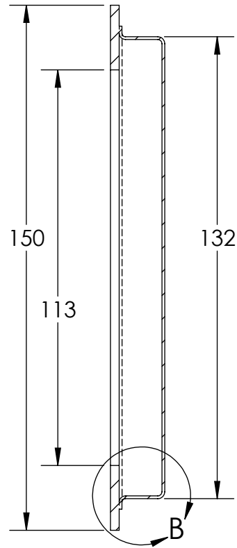
SECTION A-A
