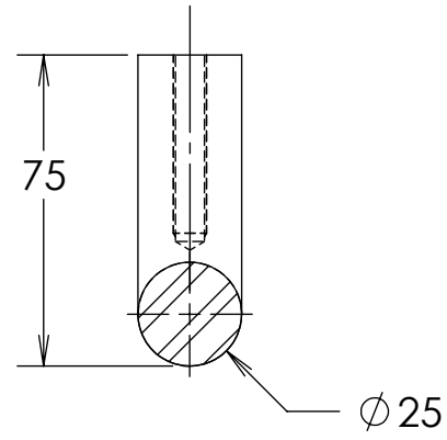
8210-25 A-A
