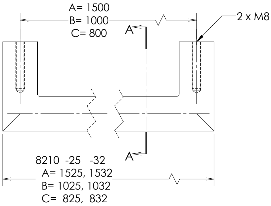
8210-32 A-A
