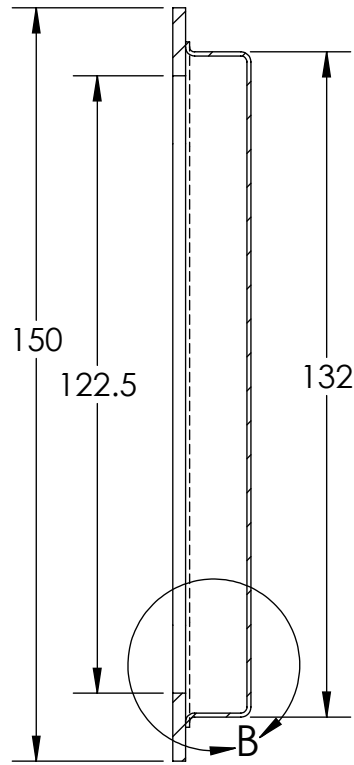
SECTION A-A
