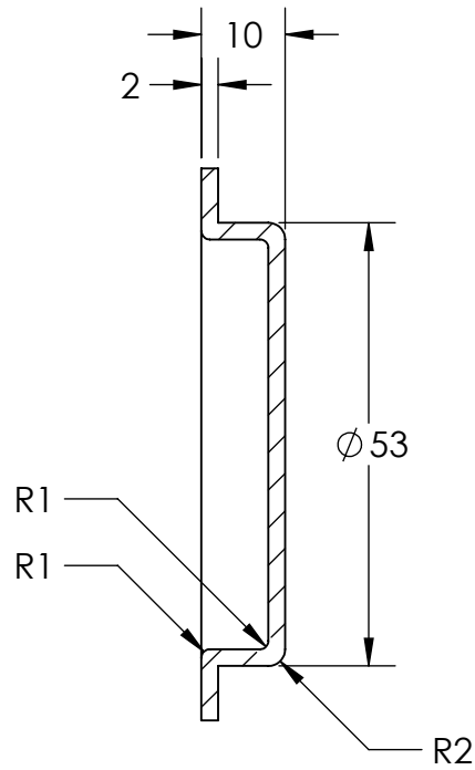
SECTION A-A
